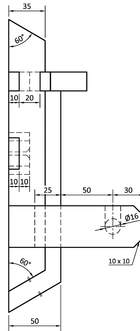
End View/Taobhchló
